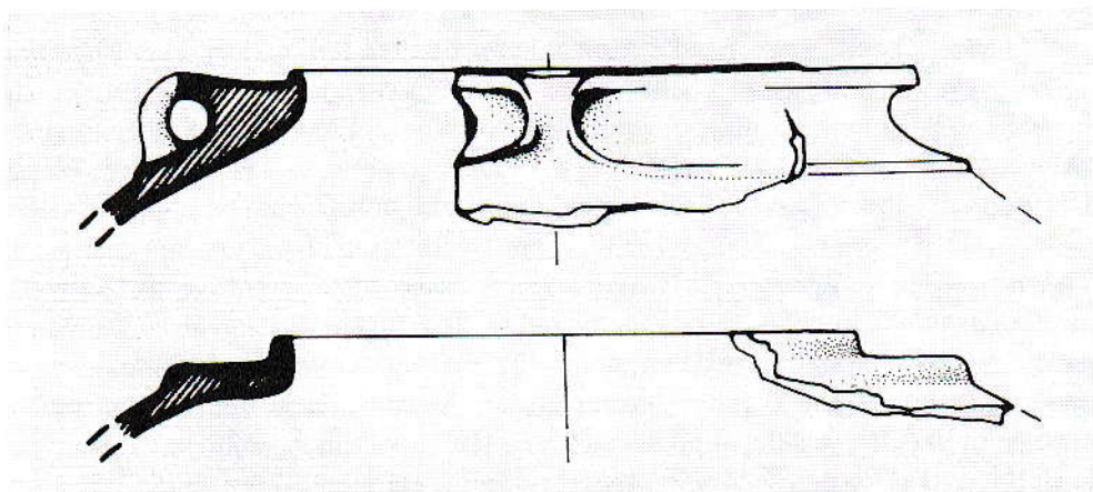
Bronastodobna lončenina iz spodnje naselbine (merilo 1:2) (Moretti 1978)
